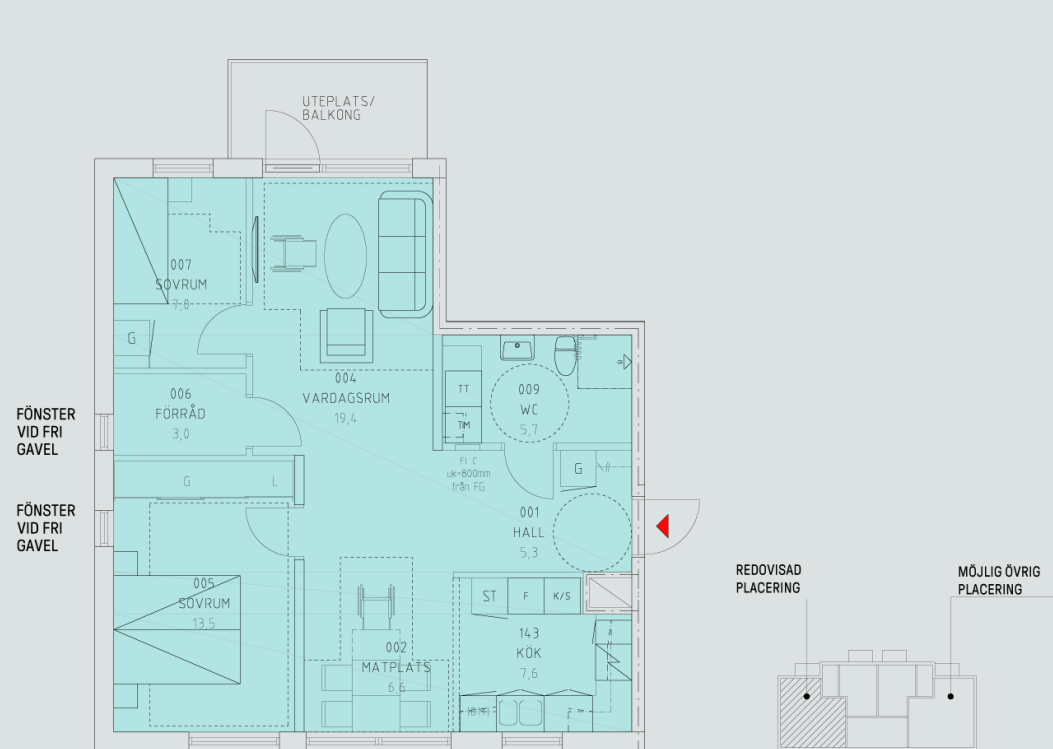
PLANLÖSNING 3RoK 70,0 m 2 PLAN 1-4 I KOMBINATION MED 2RoK, SE RITNING 7
