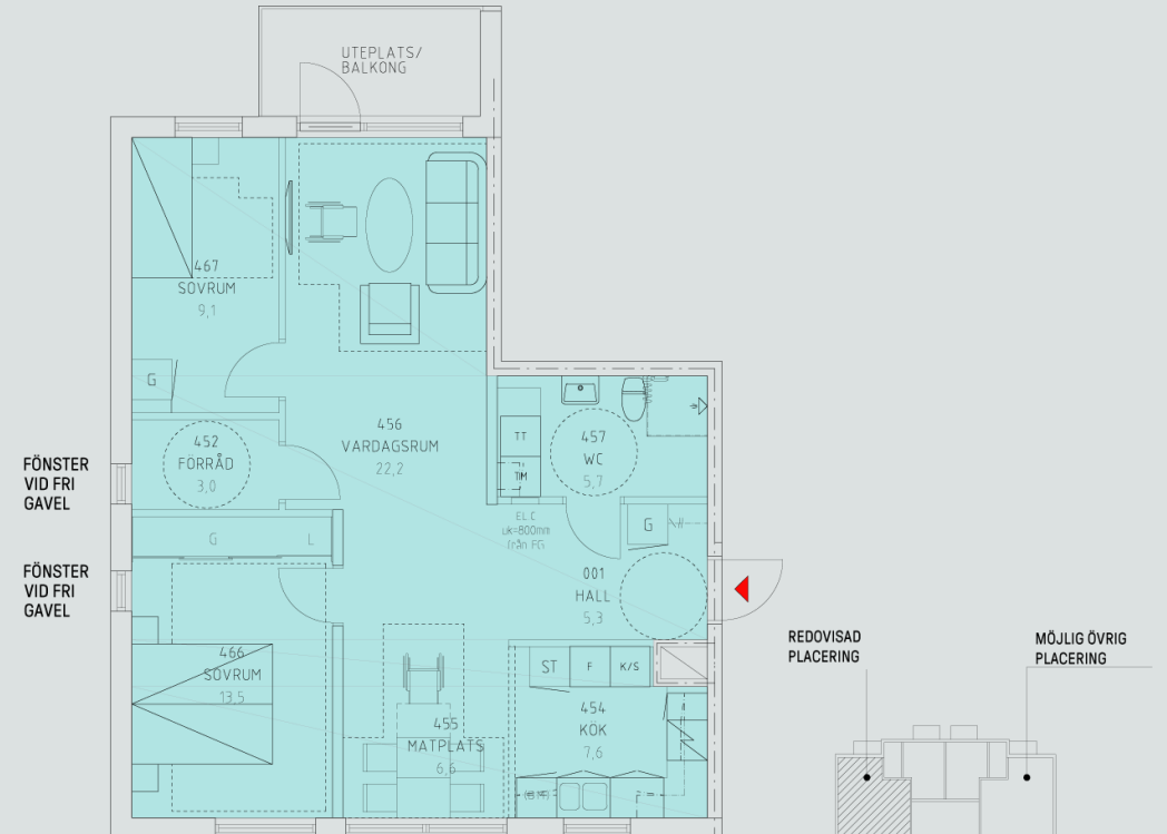
PLANLÖSNING 3RoK 75,0 m 2 PLAN 1-4 I KOMBINATION MED 2RoK, SE RITNING 7
