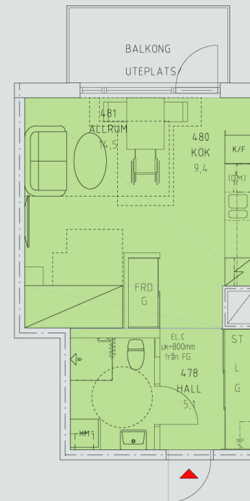
ALTERNATIV PLANLÖSNING 1RoK 35,6 m 2 PLAN 1-4 I KOMBINATION MED 4RoK, SE RITNING 9
