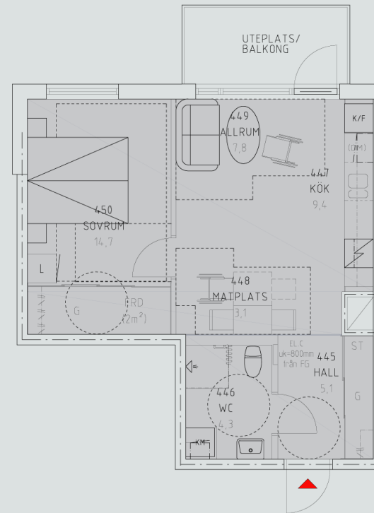
PLANLÖSNING 2 RoK 45 m 2 PLAN 1-4 I KOMBINATION MED 3ROK, SE RITNING 8
