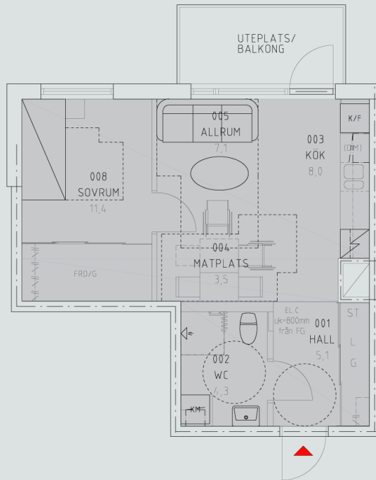
PLANLÖSNING 2 RoK 39,9 m 2 PLAN 1-4 I KOMBINATION MED 3ROK, SE RITNING 8
