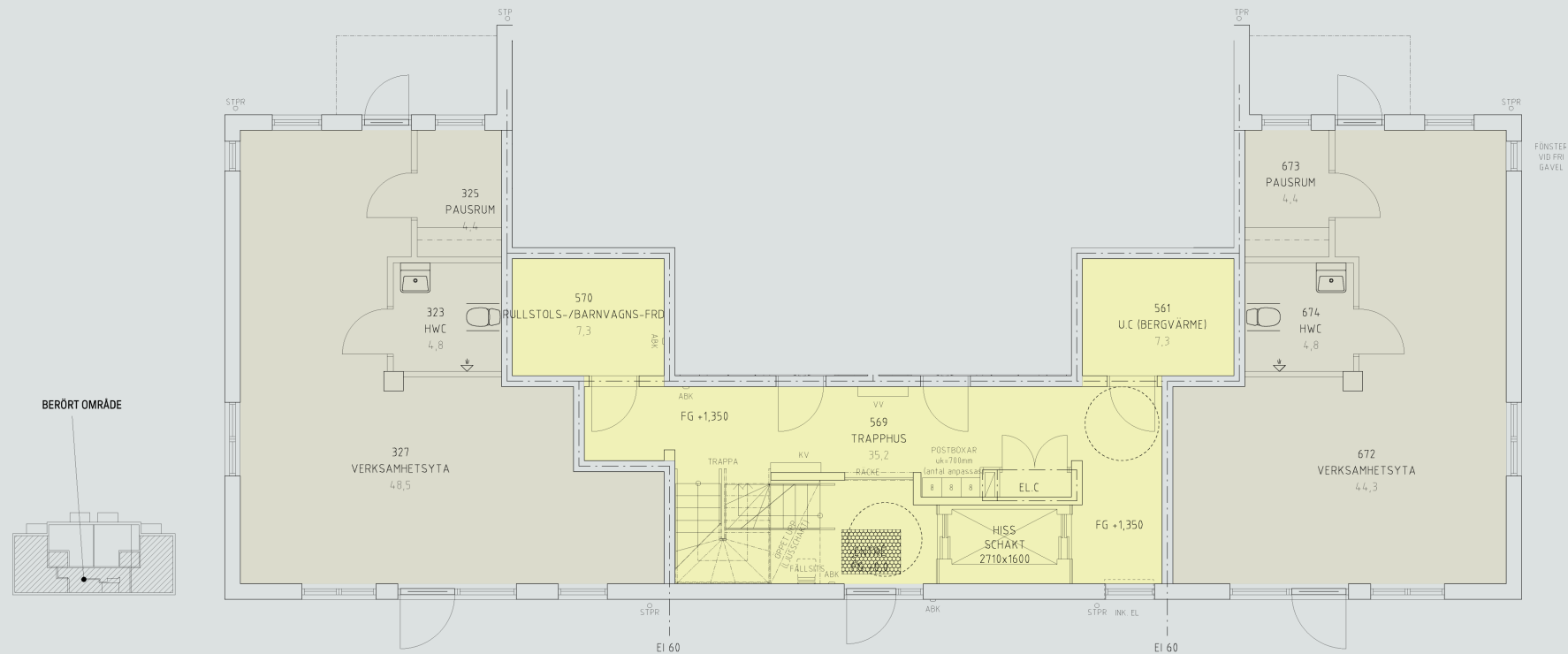
OPTION - FÖRHÖJD VÄNINGSHÖJD (PÅ DEL AV BOTTENPLAN)
